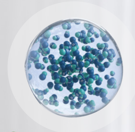
Vees sisalduvad hüdroksüülradikaalid
